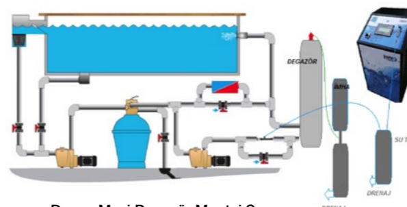
Dozon Maxi Degazör Montaj Şeması Dozon Maxi Degastor Assembly Diagram
